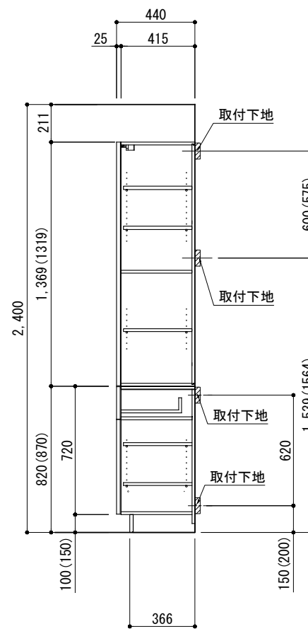
B面展開図
