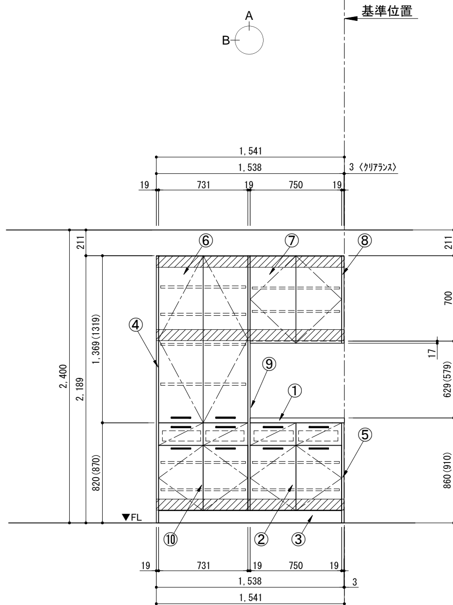
A面展開図
