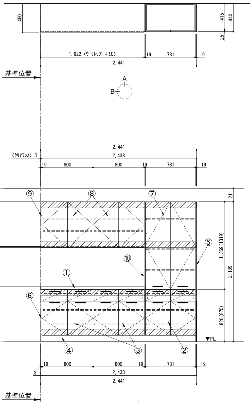
A面展開図
