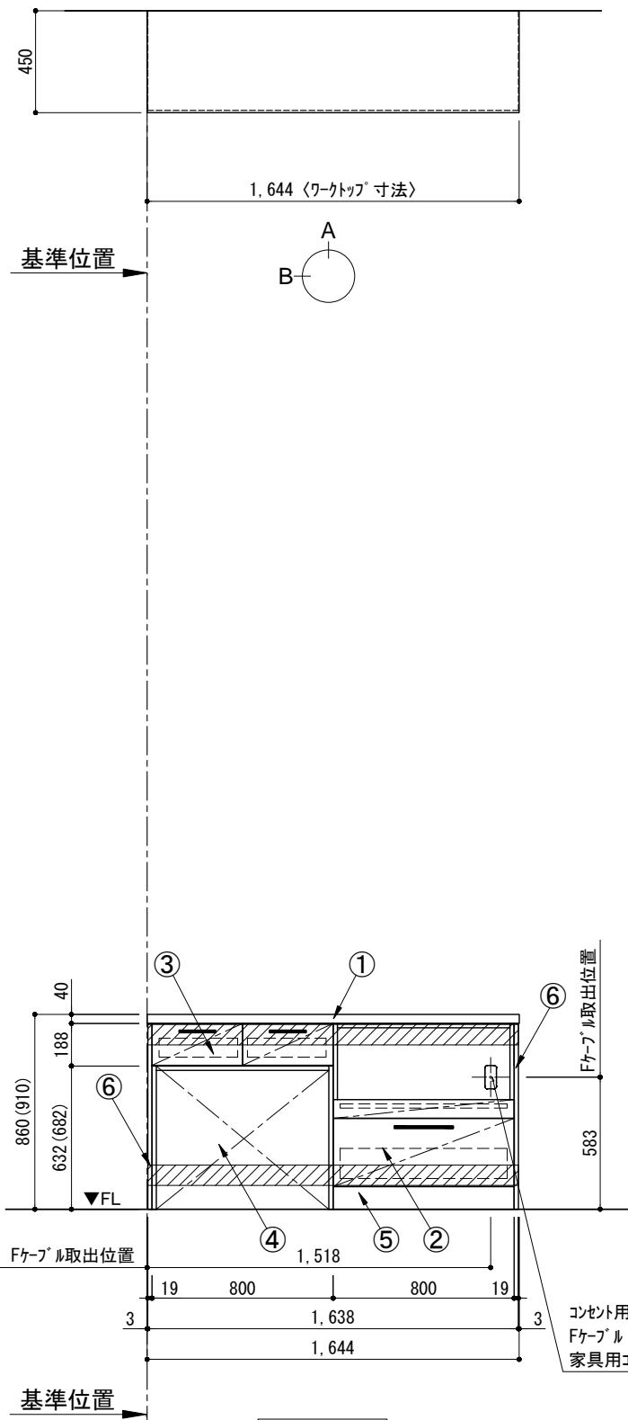
A面展開図
