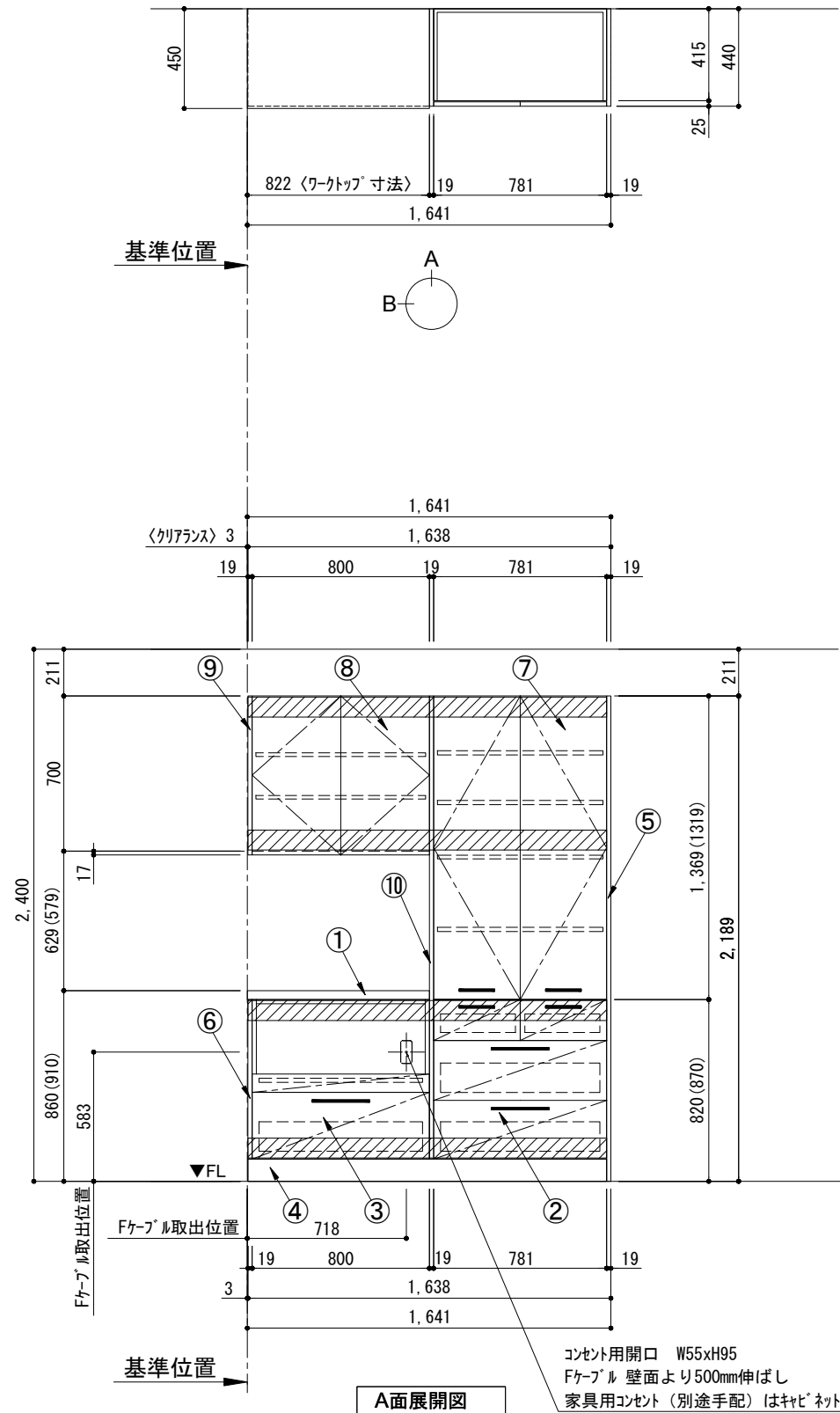
A面展開図
