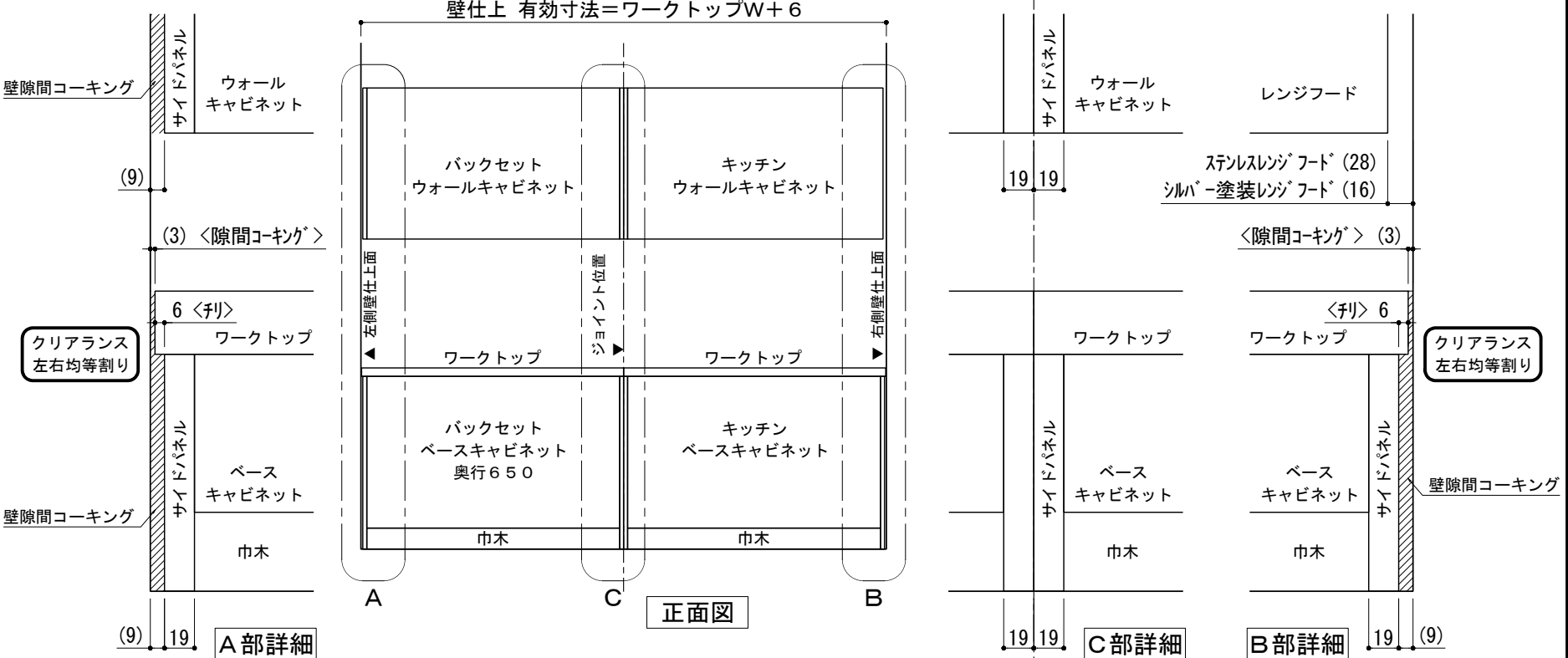
④ 横並び設置×両側側面壁 納まり
