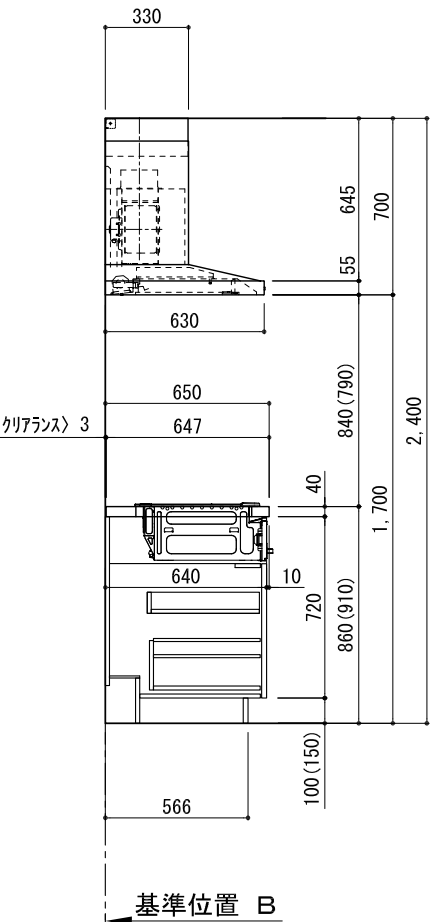
A面展開図
