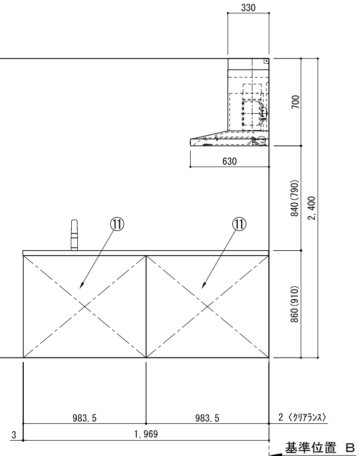
C面展開図
