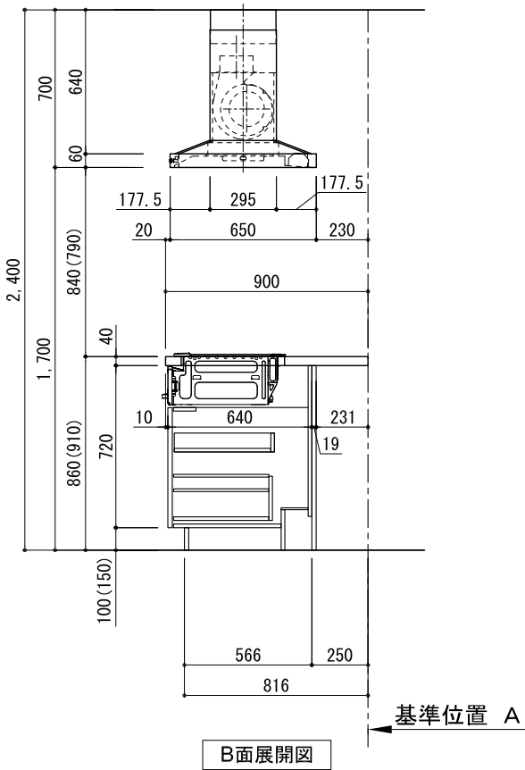
C面展開図
