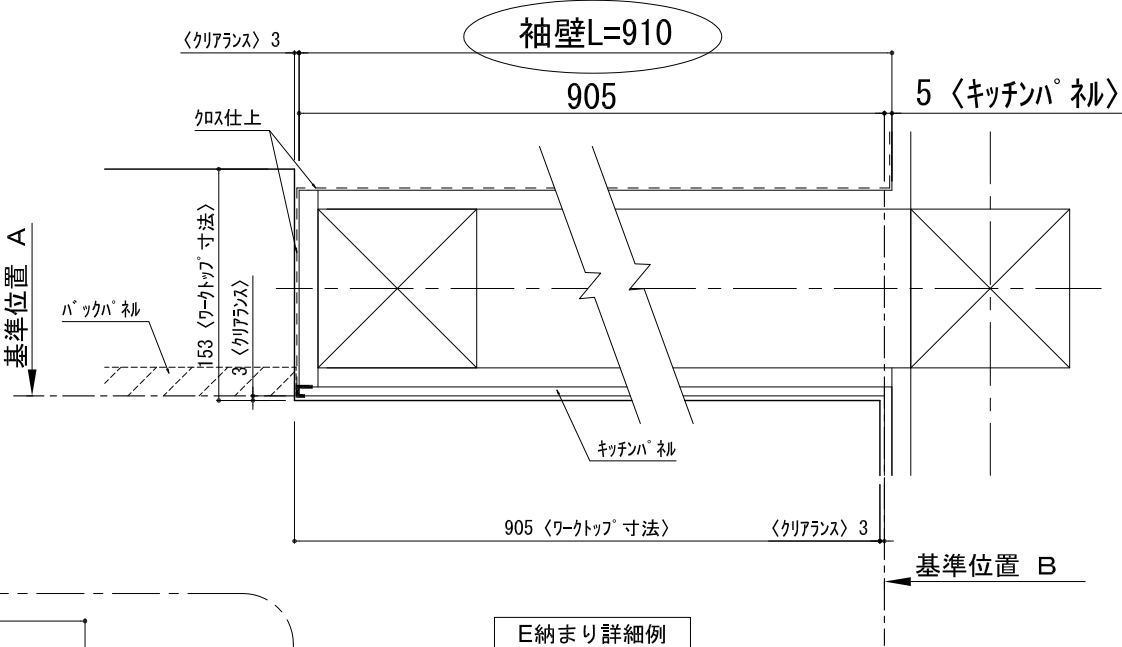
E納まり詳細例
