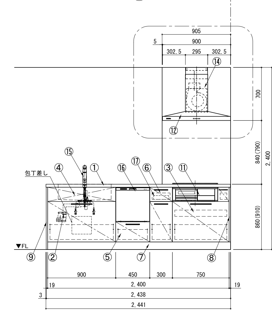
A面展開図
