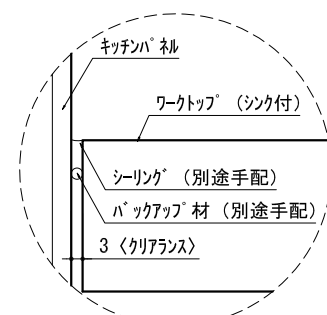
F 詳細図
