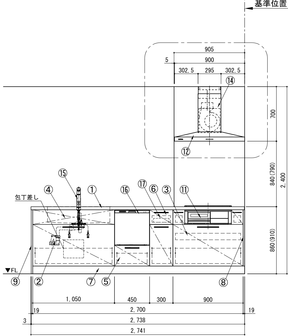
A面展開図
