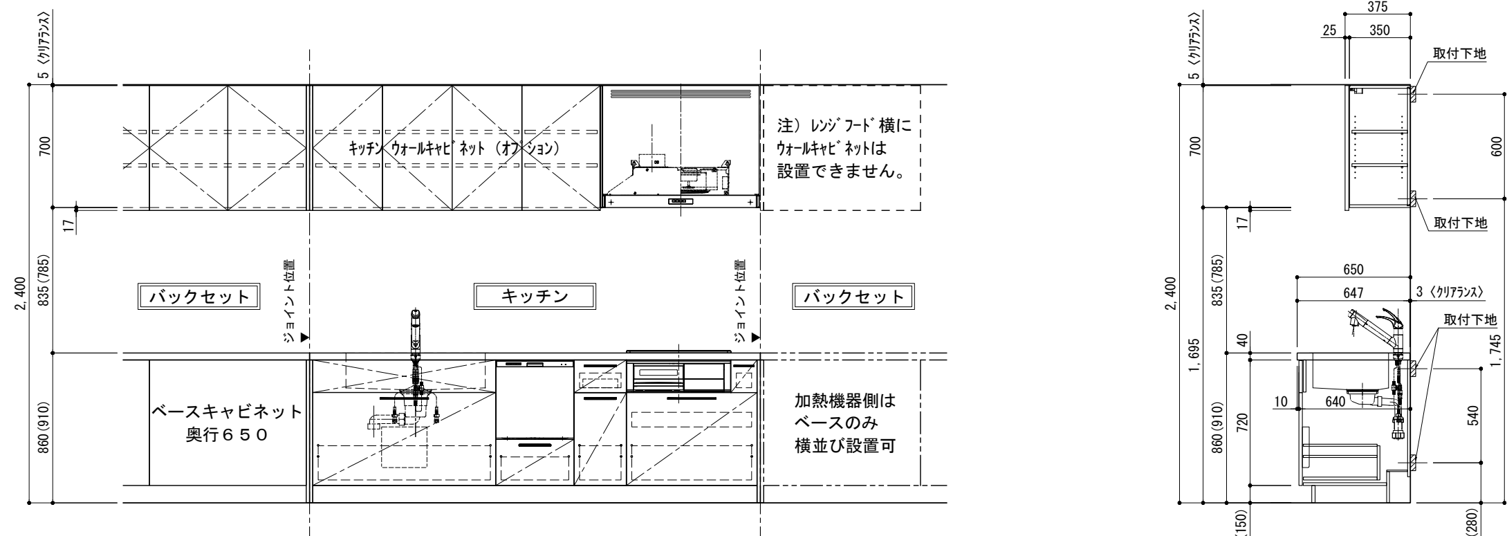
シルバー塗装レンジフード用ウォールキャビネット（Bタイプ）取付高さ
