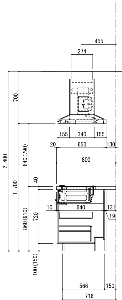
B面展開図
