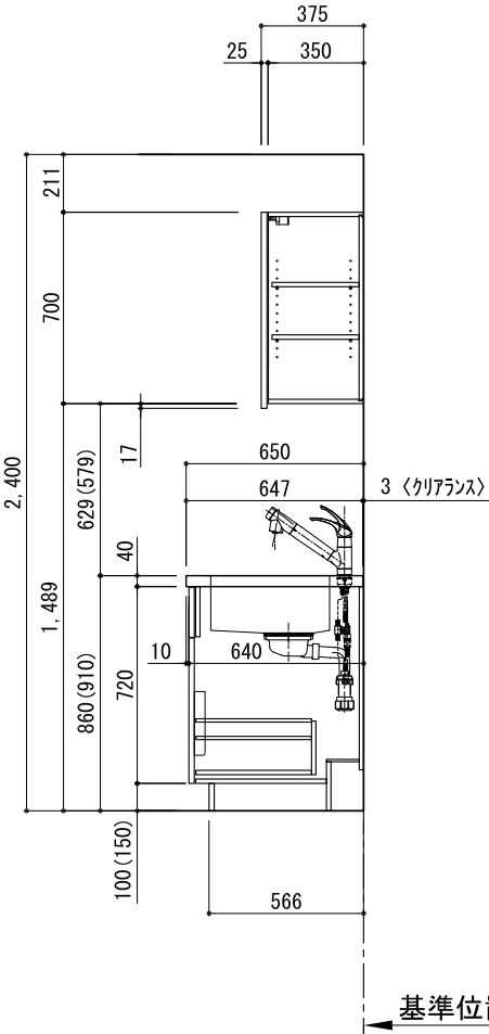
B面展開図
