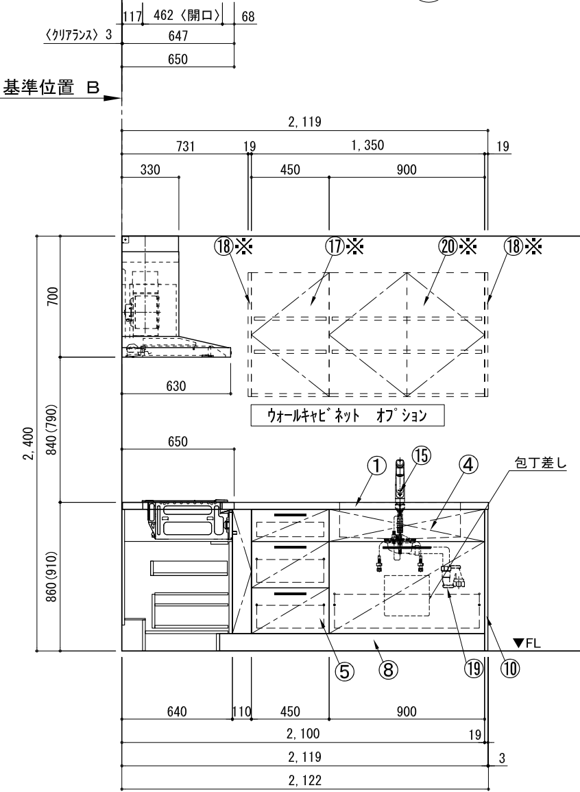
A面展開図
