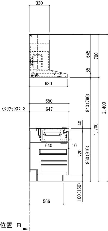
A面展開図
