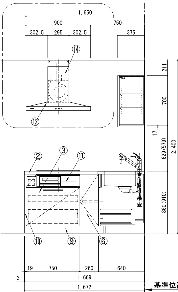
B面展開図
