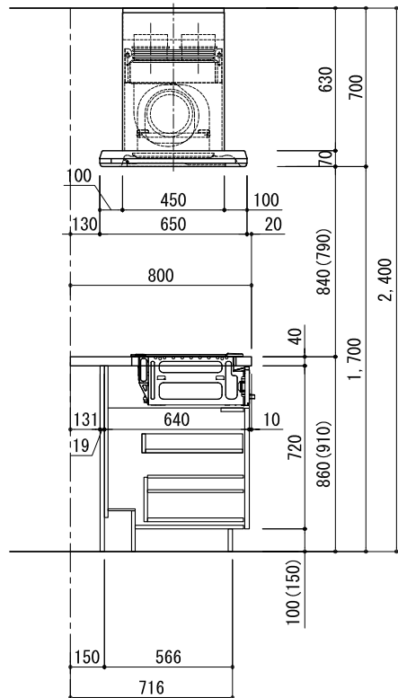
C面展開図
