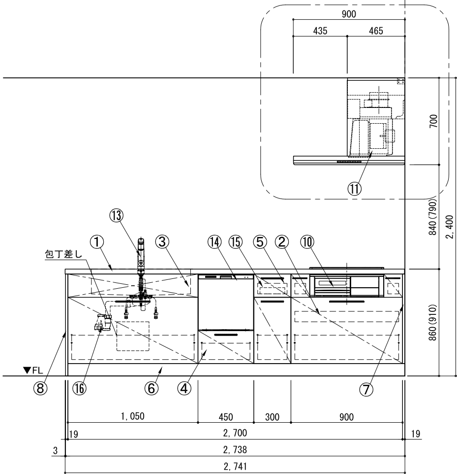
A面展開図
