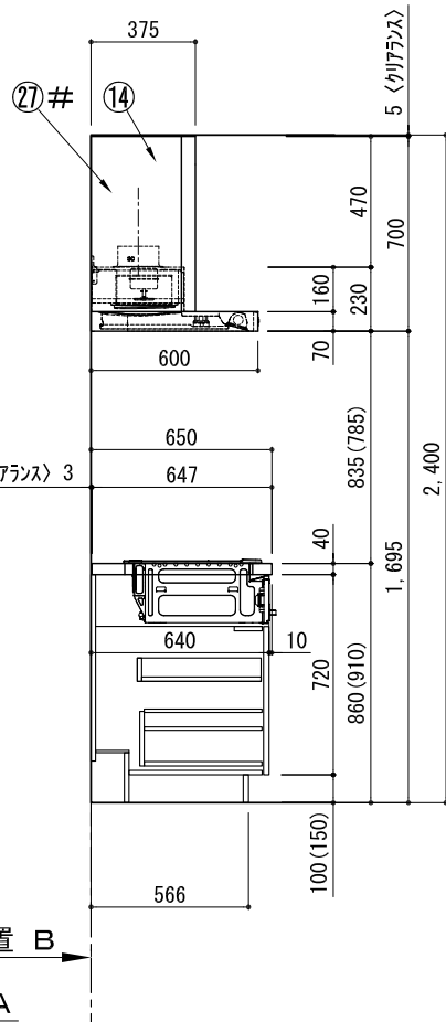
A面展開図
