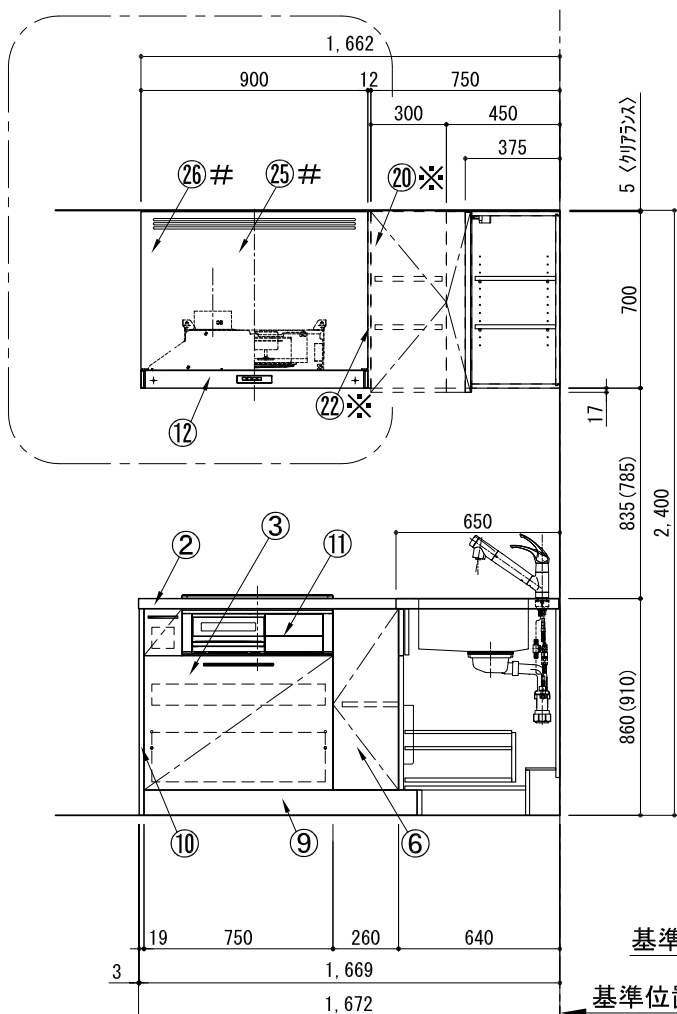
B面展開図
