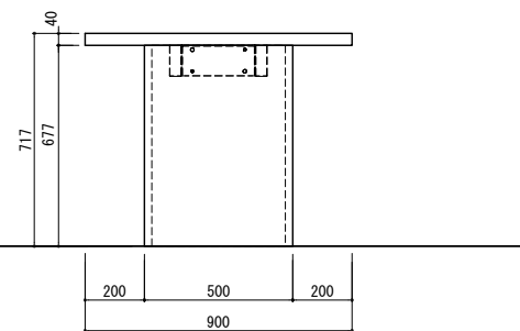
B面展開図
