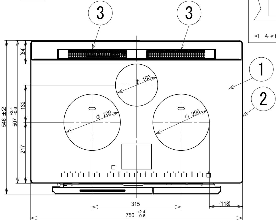
平面図
