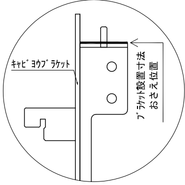
▼ボックスラック 設置位置拡大図
